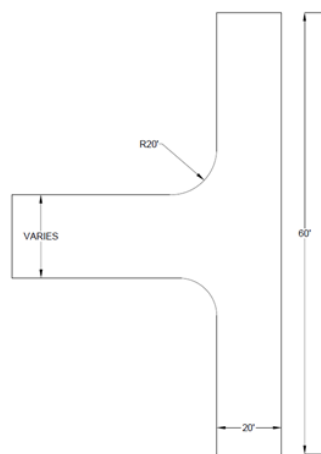
HAMMERHEAD (D)
